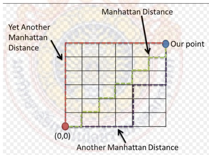
ภาพที่ 2.8 แสดงระยะทางแบบ Manhattan Distance
