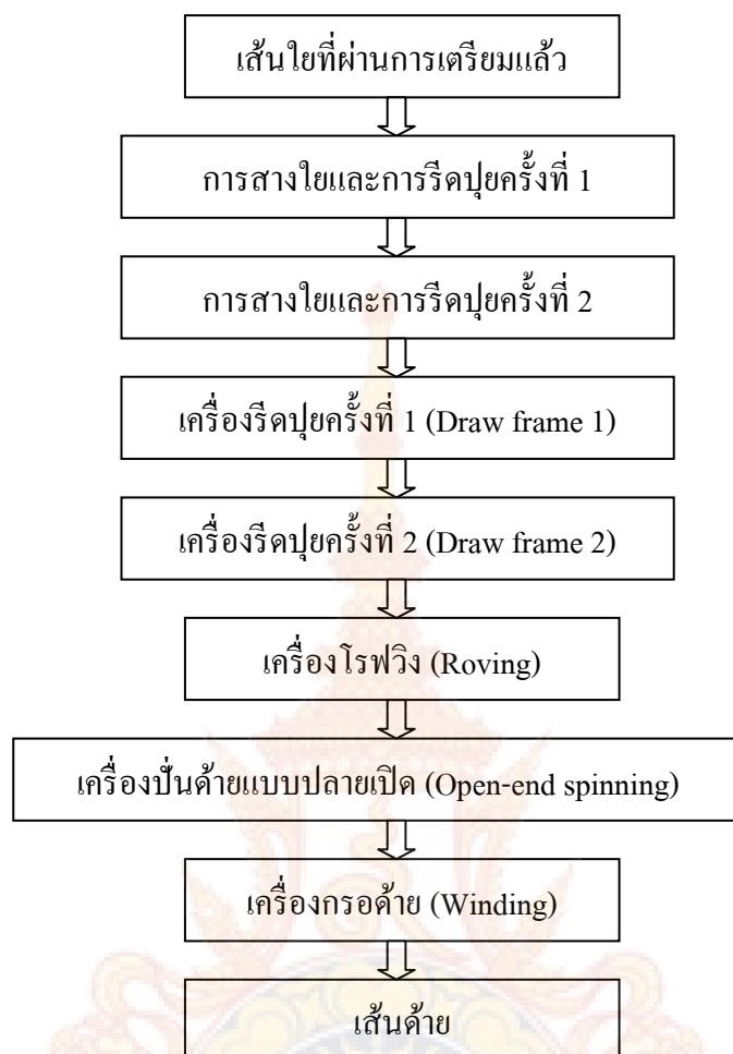
ภาพที่ 3.1 กระบวนการปั่นด้ายแบบปลายเปิด
