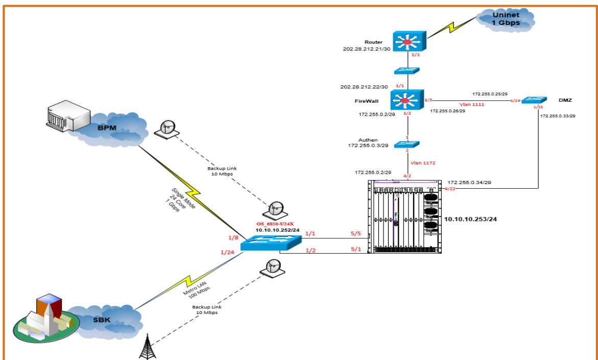
รูปภาพแสดง โครงข่ายสำรอง (Backup Link)
