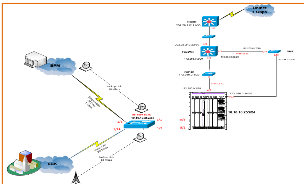
รูปภาพแสดง โค้งขายสำรอง (Backup Link)
